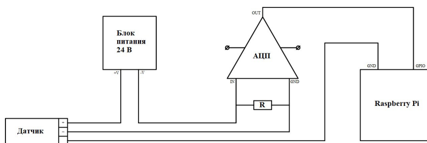
Рис. 5. Схема подключения датчика давления
