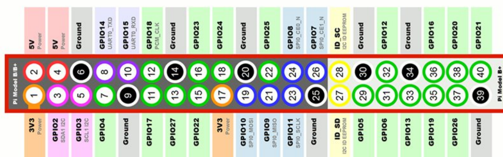
Рис. 16. Распиновке микроконтроллера
