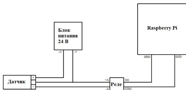
Рис. 9. Схема подключения концевого датчика
